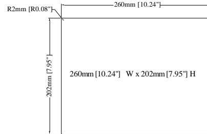
Cutout Dimensions
