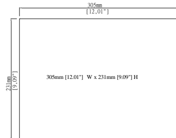
Cutout Dimensions
